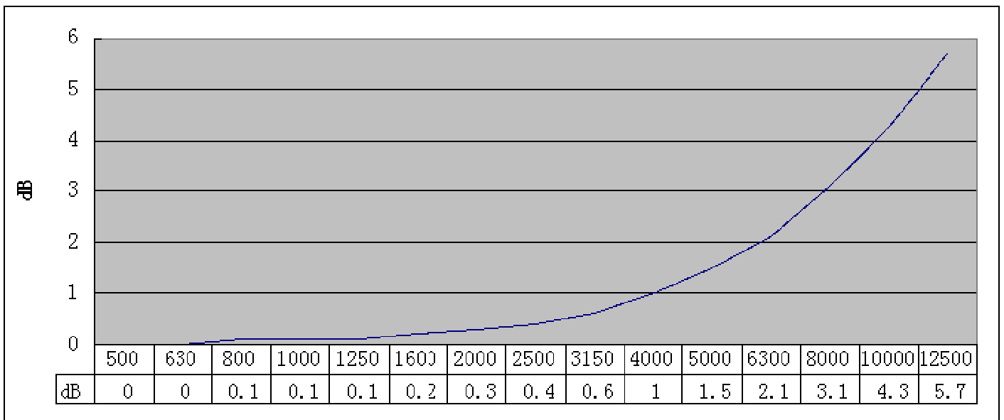
指向设为 90° 时的 Z 计权响应
